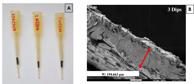
Figura 2. Unidades de extracción preparadas con el papel recubierto de SWNHs (A). Imagen SEM del recubrimiento (B). Reproducida bajo licencia Creative Commons de la referencia [4]
