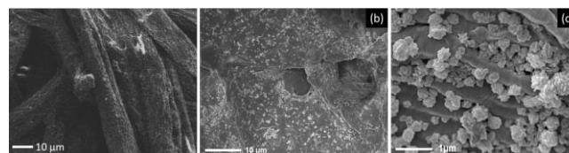
Figura 3. Imágenes SEM del papel recubierto con Nylon 6 y AgNFs a distintos aumentos.
