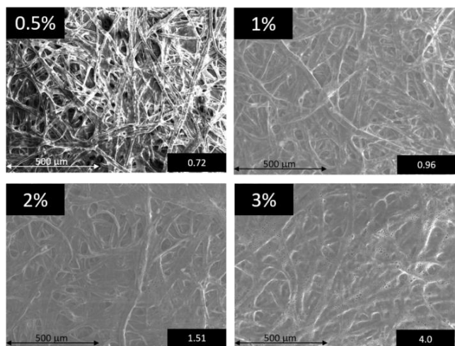
Figura 1. Imágenes SEM del recubrimiento del papel con distintos porcentajes de poliestireno. Reproducida de la referencia [3] con permiso de Elsevier.
